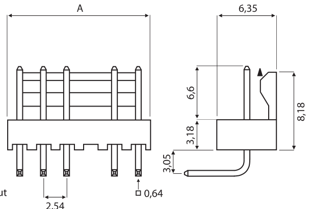
Stiftleiste gewinkelt
