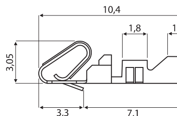
Buchsenkontakt
