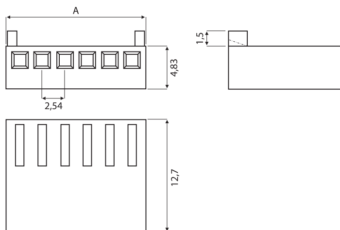
Buchsengehäuse
