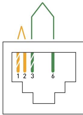
T568B
