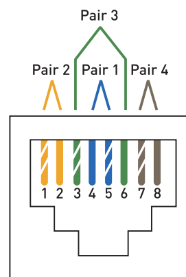
T568B
