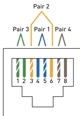
T568A
