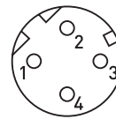
Polbild M12 D-kodiert (Steckseite Gerätedose)
